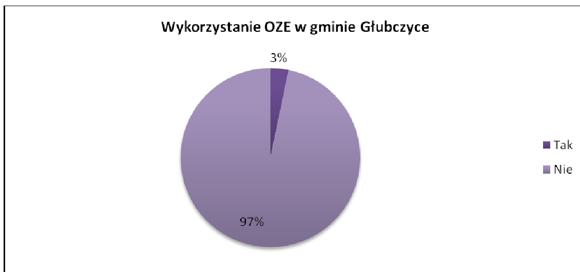
Wykres 8 Wykorzystanie instalacji OZE lub ze źródła ekologicznego w gminie Głubczyce (źródło: opracowanie własne na podst. ankiet).
