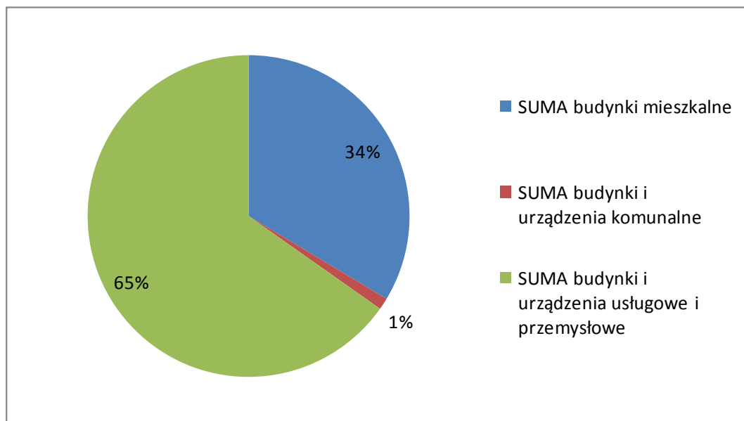
Wykres 23 Procentowy wykres zużycia energii w roku prognozowanym - 2020 w Gminie (źródło: opracowanie własne na podst. danych od PGNiG)
