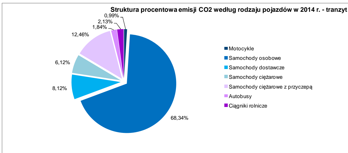
Wykres 18 Emisja CO 2 z tranzytu w 2014 według rodzaju pojazdów (źródło: opracowanie własne na podst. danych z CEPIK-u i GDDKiA)
