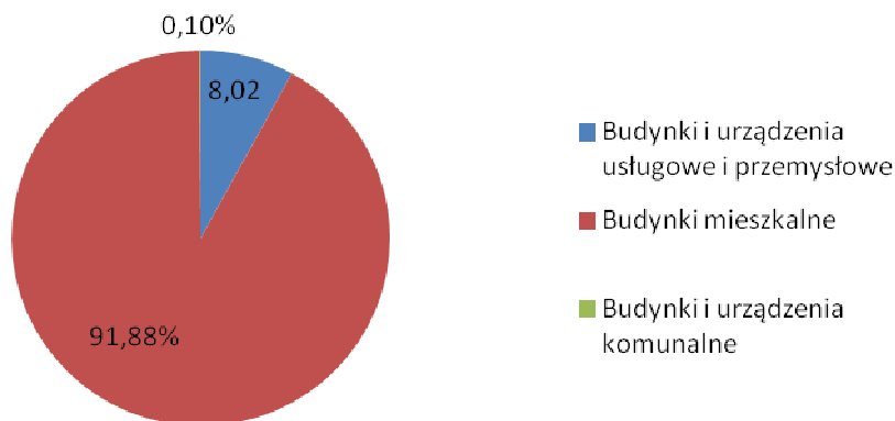
Wykres 13 Emisja CO 2 z ogrzewania w 2014 roku według sektorów (źródło: opracowanie własne na podst. ankiet).
