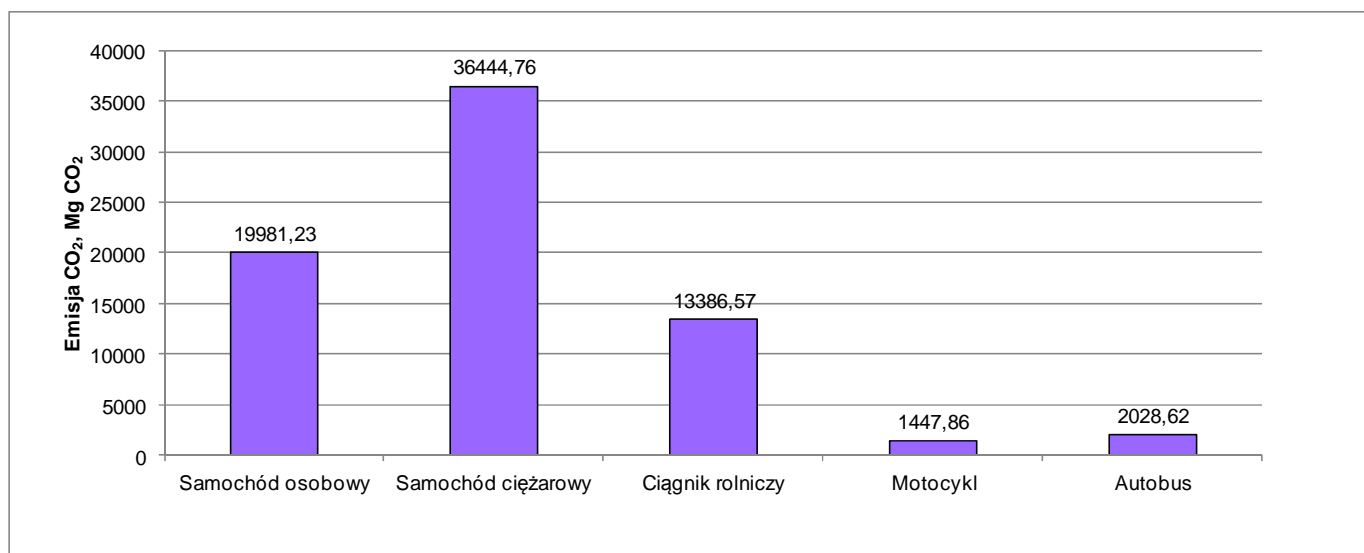
Wykres 14 Emisja CO 2 z transportu lokalnego według rodzaju pojazdów w 2014 roku (źródło: opracowanie własne na podst. danych z CEPIK-u)
