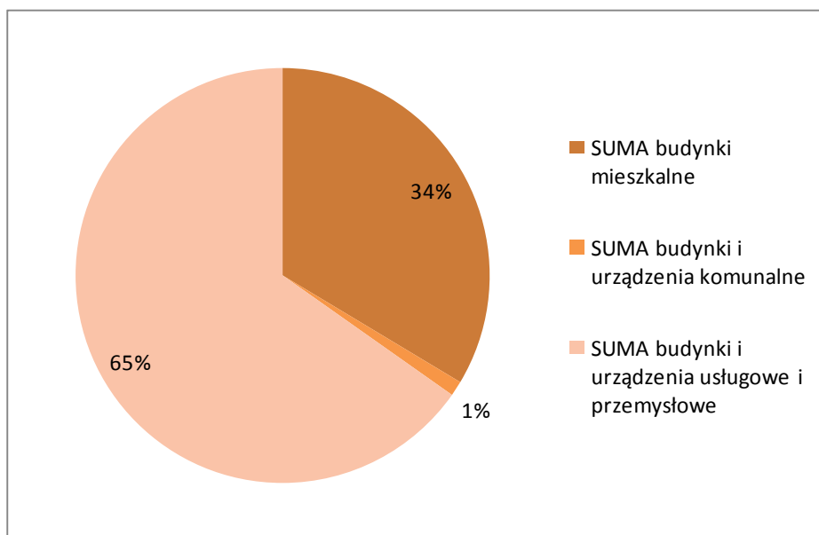
Wykres 20 Struktura emisji CO 2 związana ze zużyciem gazu w roku 2014 (źródło: opracowanie własne na podst. danych od PGNiG)
