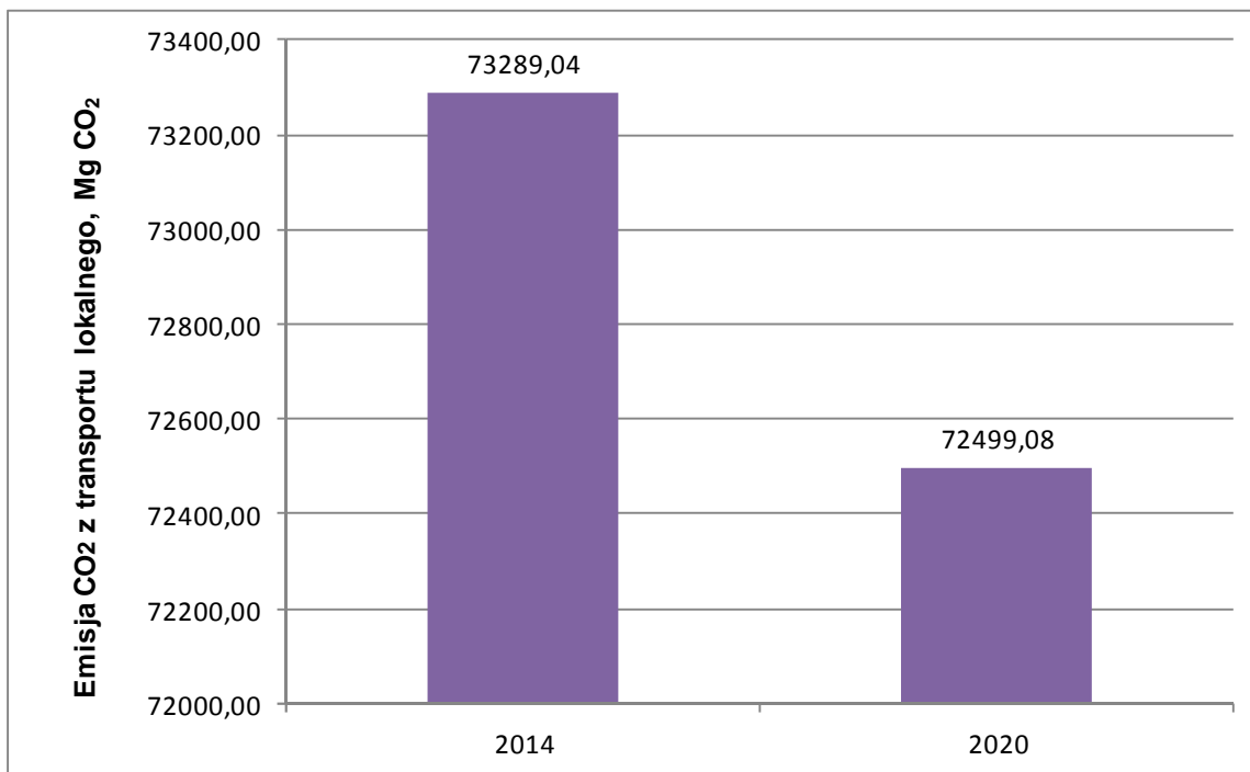
Wykres 16 Emisja CO 2 z transportu lokalnego w roku bazowym - 2014 i prognoza na rok 2020 (źródło: opracowanie własne na podst. danych z GDDKiA)
