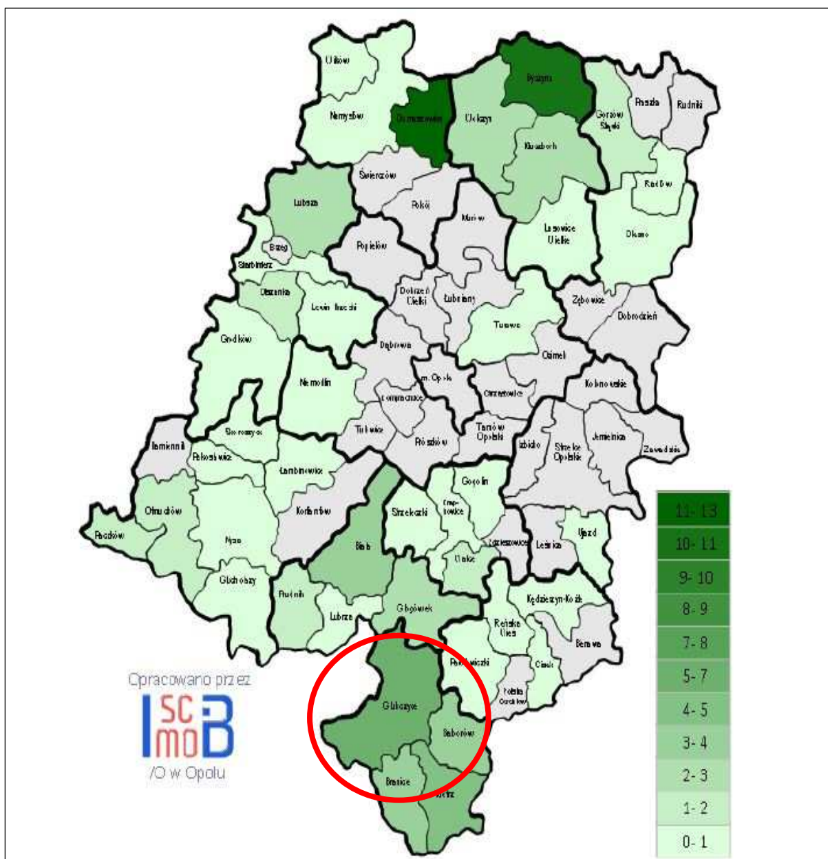
Rysunek 5 Potencjał techniczny wykorzystania biogazu rolniczego w województwie opolskim, GWh/rok (źródło: Planu Rozwoju Odnawialnych Źródeł Energii w Województwie Opolskim)
